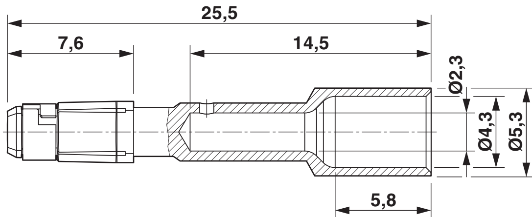
Maßzeichnung
