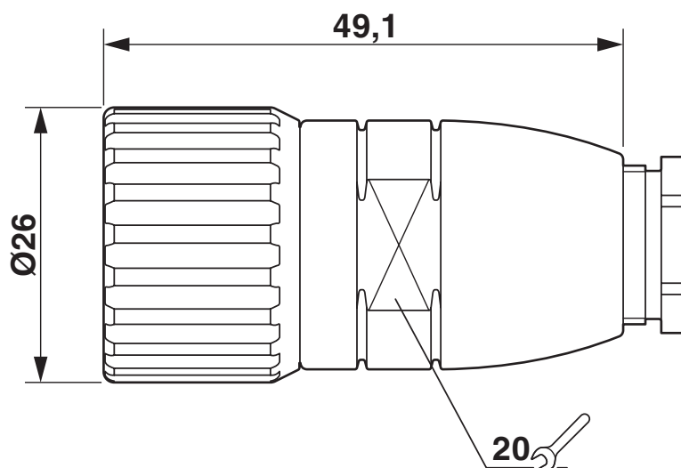
Maßzeichnung
