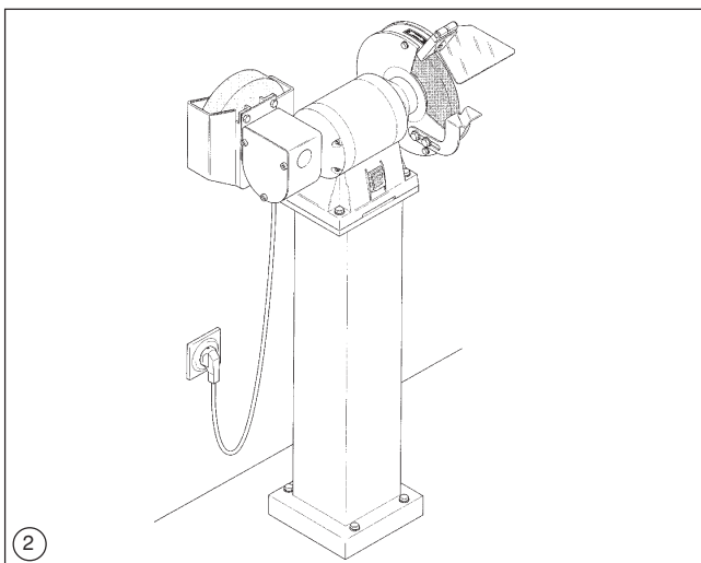
Maschinenständer Best.-Nr. 090 000 1134
