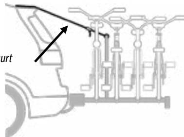
Bild 19: Zugentlastungsgurt
