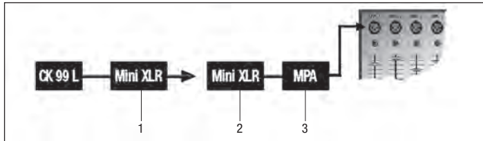
Fig. 1: Schema di collegamento con MPA V L (opzionale)
