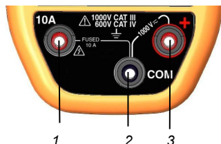
Figure 4 : les bornes
