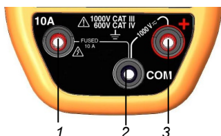
Figura 4: i morsetti
