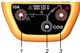
Figura 4: los terminales
