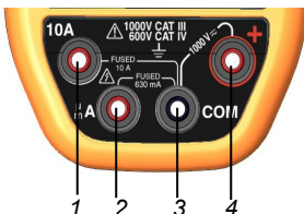
Abbildung 4: die Buchsen
