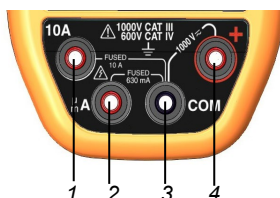
Figure 4 : les bornes
