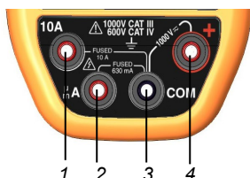
Figura 4: los terminales
