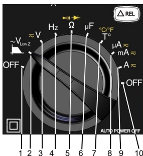
Abbildung 1: Drehschalter
