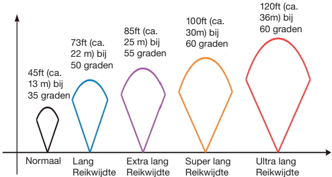
Afbeelding 6 PIR-registratiebereik
