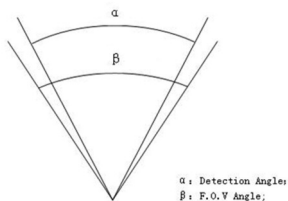
Abbildung 7 Erfassungswinkel vs. Blickwinkel
