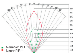
Abbildung 8 Vergleich der Erfassungsbereiche von neuen und bestehenden PIRs
