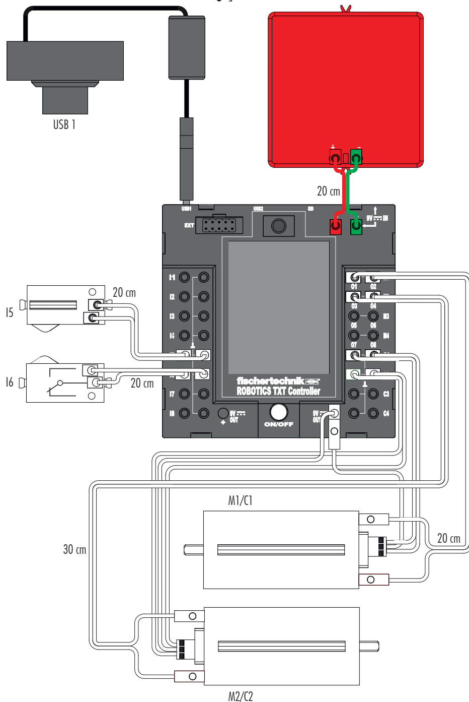
Schema elettrico Схема подключения 电路图
