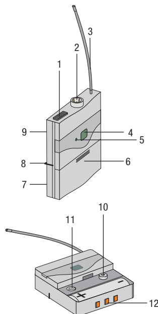
Figura 4: Controles del transmisor PT420
