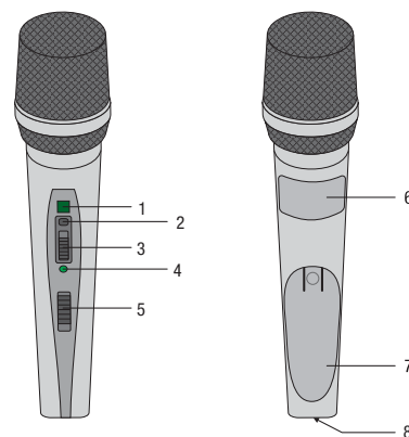
Figura 3: Elementi di comando del trasmettitore HT420
