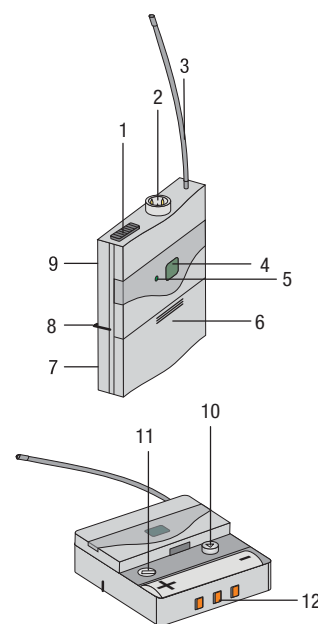
Abbildung 4: Bedienelemente des Senders PT420
