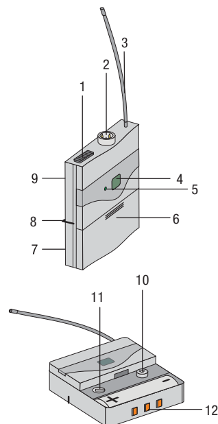
Figura 4: Dispositivos de controlo do transmissor PT420
