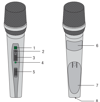
Abbildung 3: Bedienelemente des Senders HT420
