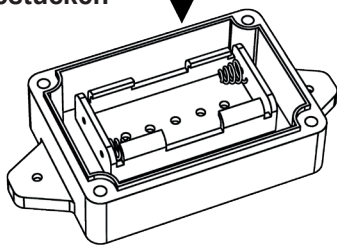
Abb. 1. Batterien Bestücken
