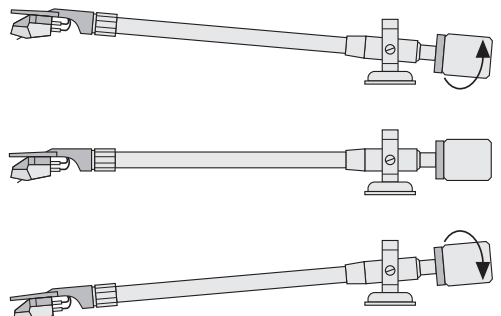
Tonarm ausbalancieren Tone arm balance ③
