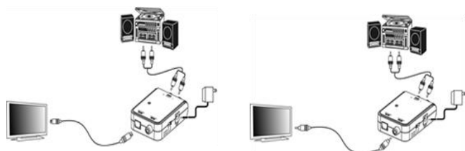
1) Conexión TOSLINK
