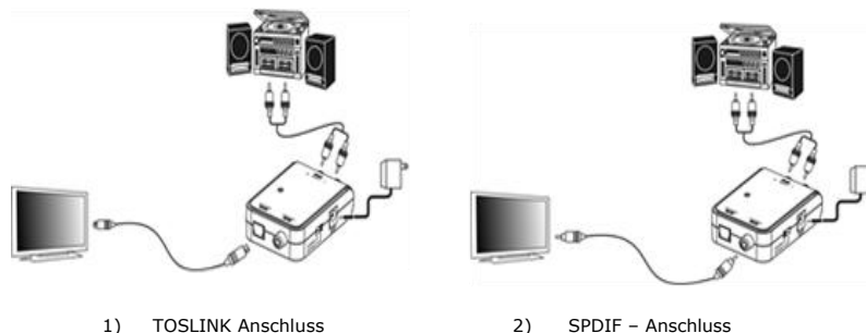
1) TOSLINK Anschluss
