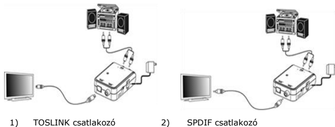
1) TOSLINK csatlakozó
