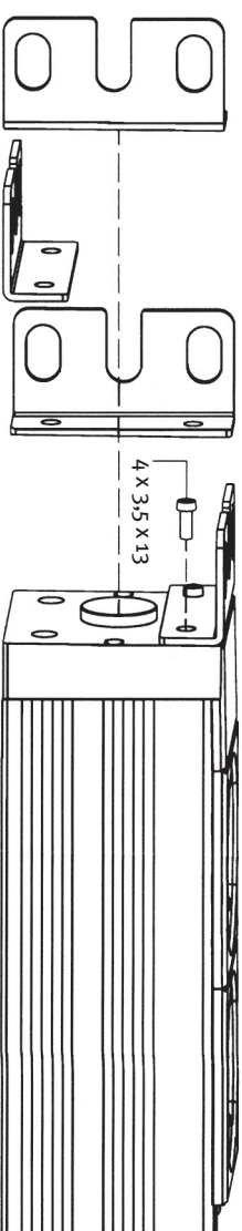
b) Blech-Befestigungswinkel / Mounting brackets of sheet metal / Equerre de fixation de lame de métal
