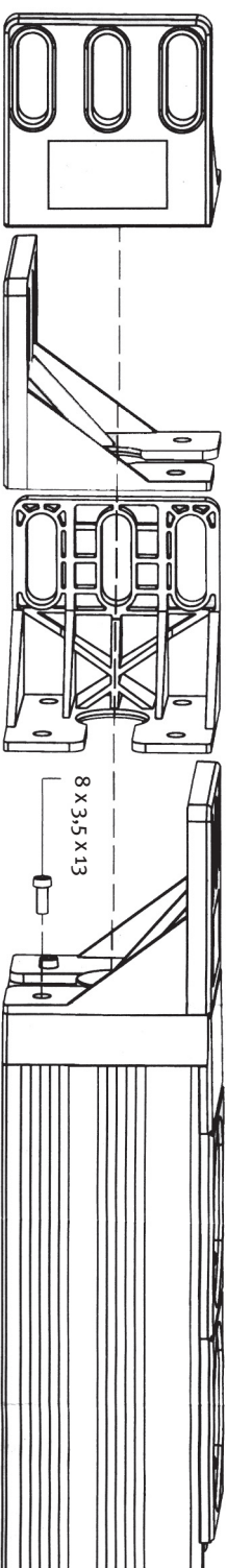
a) Kunststoff-Befestigungswinkel / Mounting brackets of plastic / Equerre de fixation de plastique
