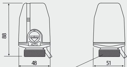
Ecrou-raccord M 30 x 1,5
