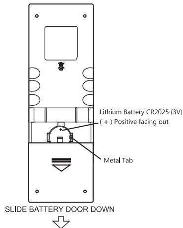
Abbildung 3. Austauschen der Batterie bei der Fernbedienung des MAC 310
