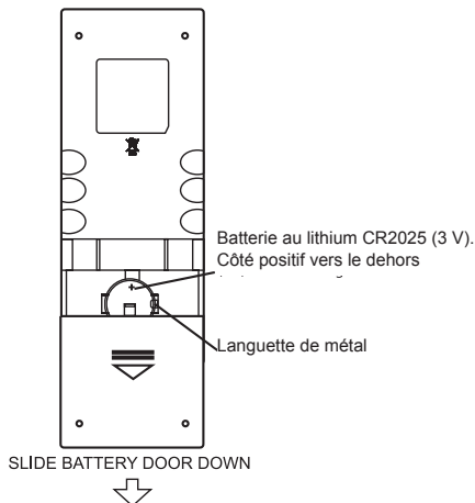
Figure 3. Changement de la batterie de la télécommande MAC 310.
