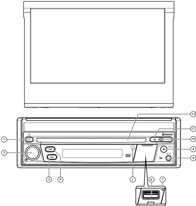
FIGURE 1. Commandes et voyants du MAC 310
