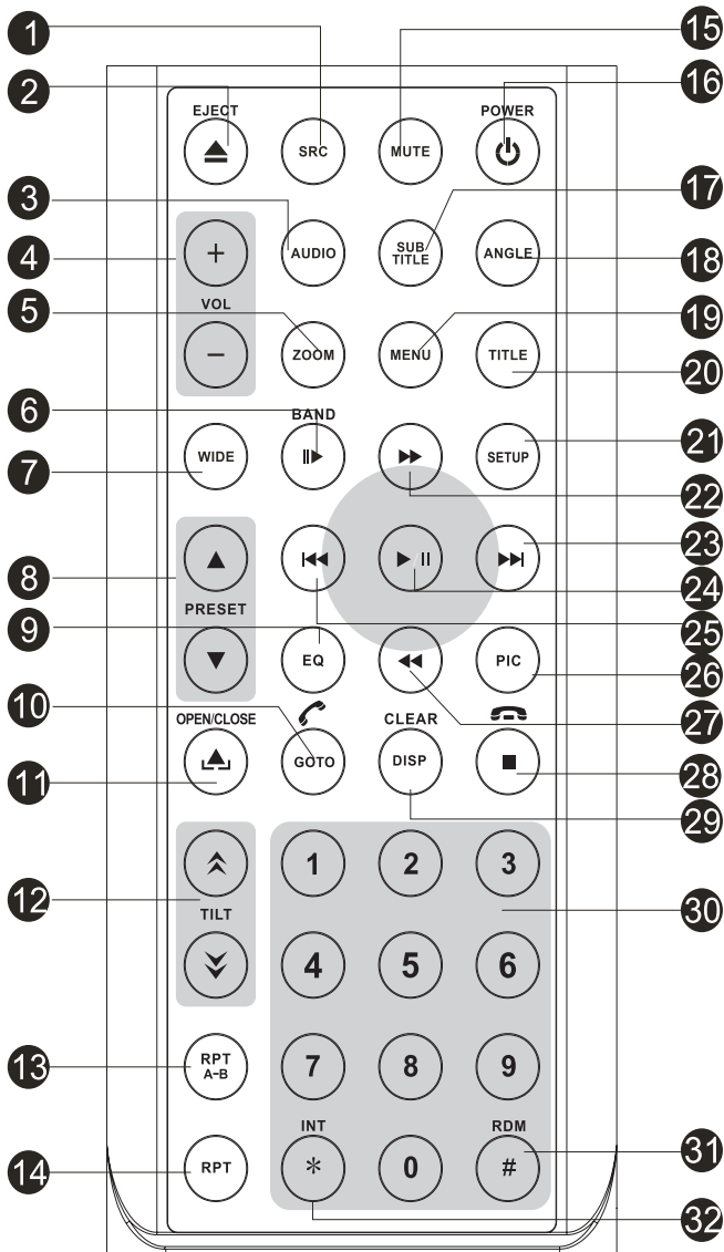
Figure 2. Télécommande MAC 310
