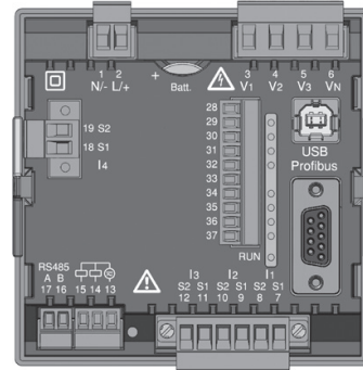
Abb. Rückseite UMG 96 RM-P (-CBM)
