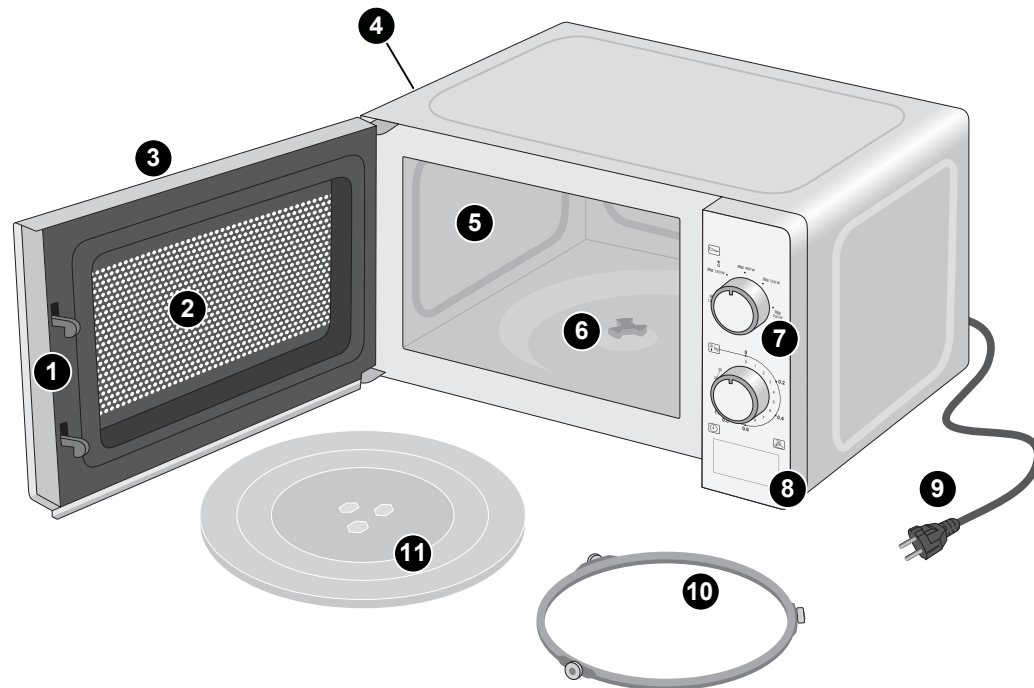
Afb. 1: Onderdelen van het apparaat
