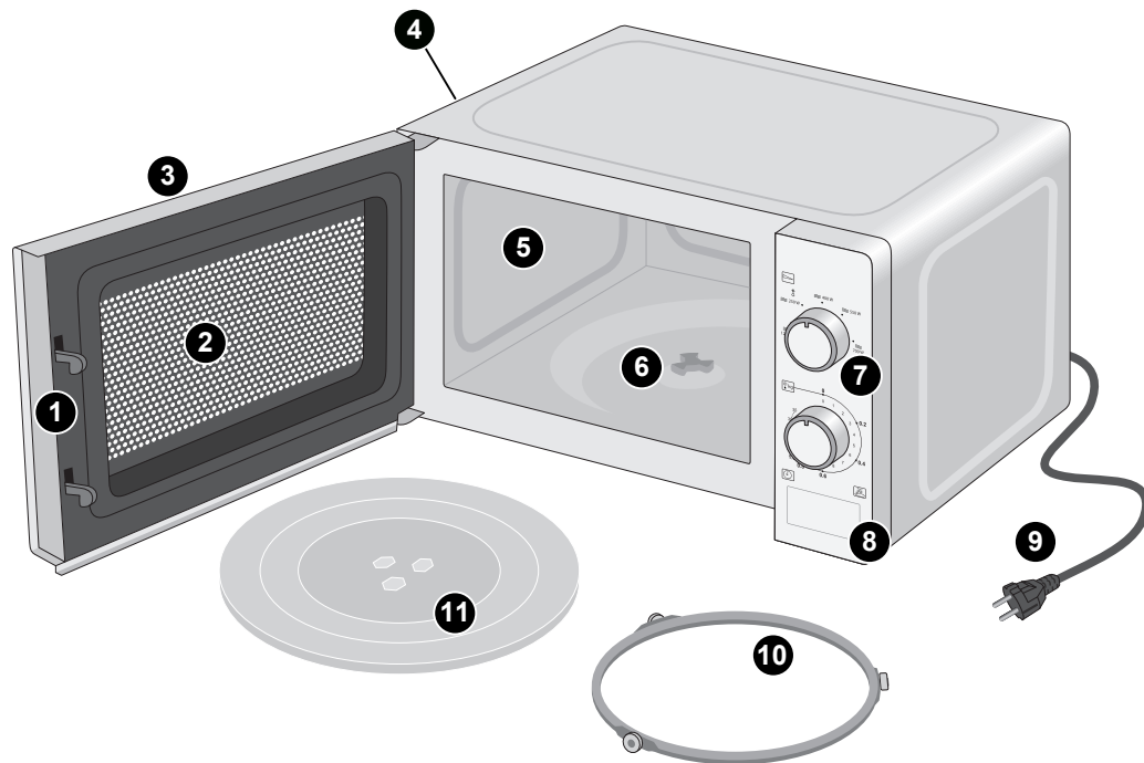
Fig. 1: Partes del aparato
