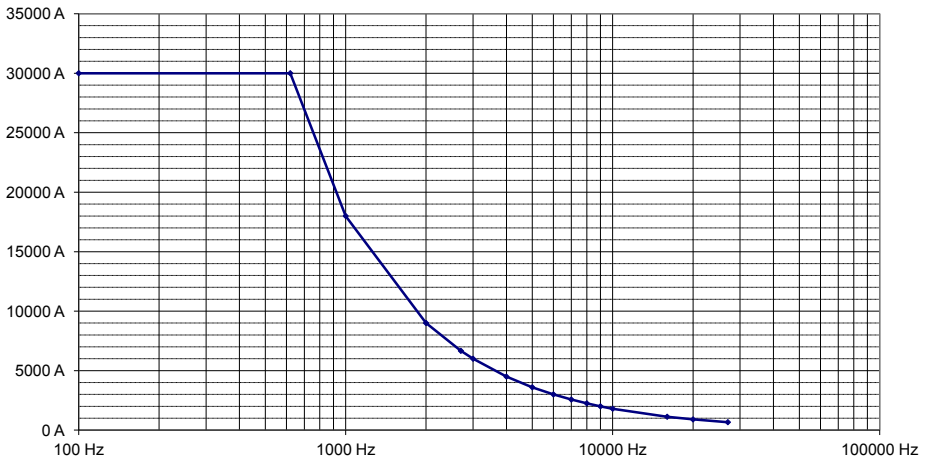
Messbereiche 30 000 A
