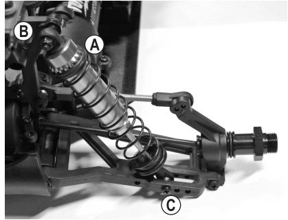
Achteras
