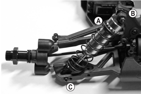
Vorderachse
