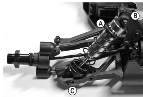
Essieu avant
