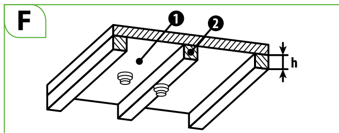
Beispiel für eine Unterteilung mit einer Höhe \leq 0,2 \text{ m}
