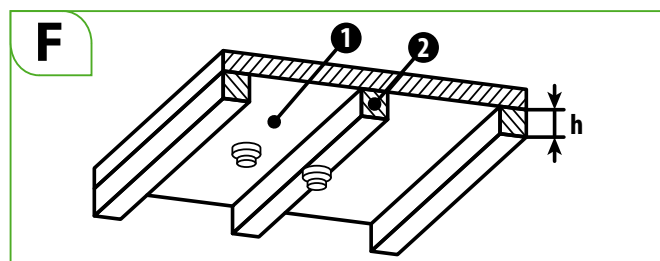
Esempio di una ripartizione a un'altezza \leq 0,2 \text{ m}
