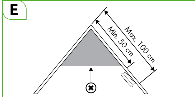
Beispiel für Unterteilungen mit einer Höhe > 0,2 \text{ m} und Deckenfeld \leq 36 \text{ m}^2
