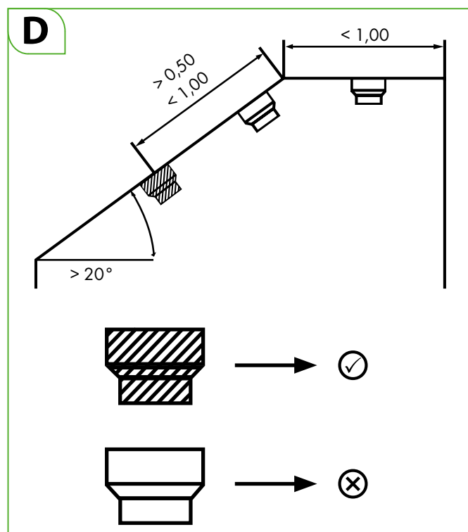
Esempio di una ripartizione a un'altezza \leq 0,2 \text{ m}
