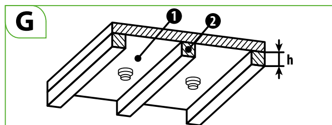
Esempio di ripartizioni con un'altezza > 0,2 \text{ m} e trave > 36 \text{ m}^2
