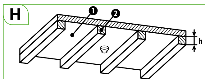
Esempio di ripartizioni con un'altezza > 0,2 \text{ m} e trave \leq 36 \text{ m}^2
