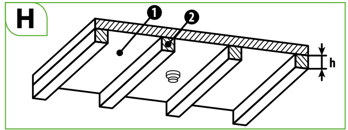
Beispiel für Unterteilungen mit einer Höhe > 0,2 \text{ m} und Deckenfeld \leq 36 \text{ m}^2
