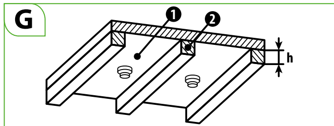
Beispiel für Unterteilungen mit einer Höhe > 0,2 \text{ m} und Deckenfeld > 36 \text{ m}^2
