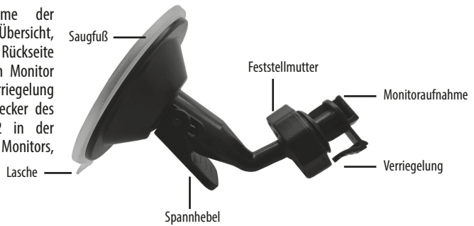
Bild 7: Monitorhalterung
