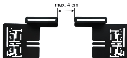
Afb. 3: Afstand camerahouders
