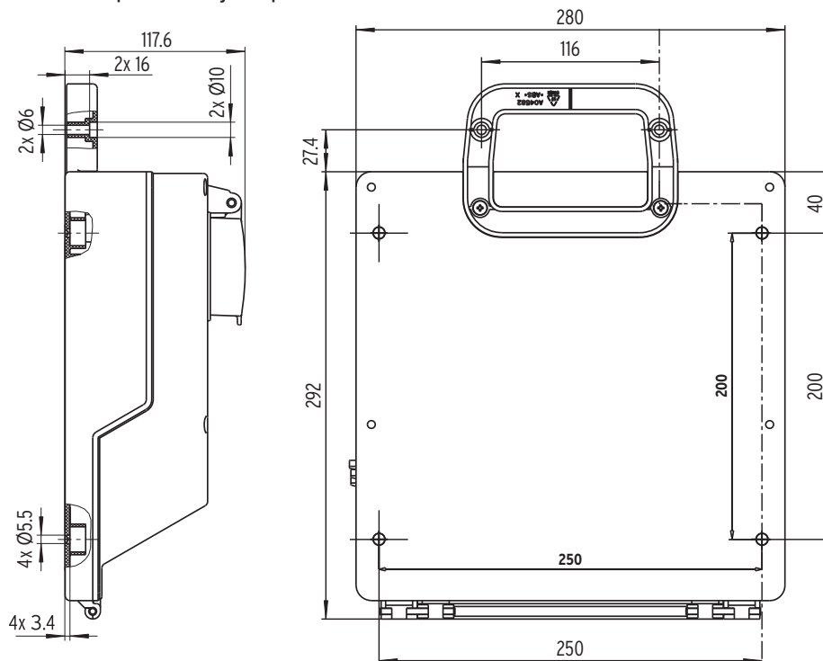
Kuva C: Poran mitat
