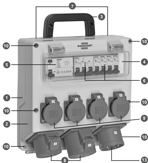
Afb. A: Voorbeeld wandverdeler 32A
