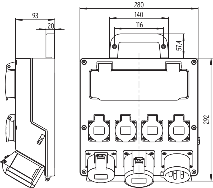
Fig. D: Dimensiones de la carcasa
