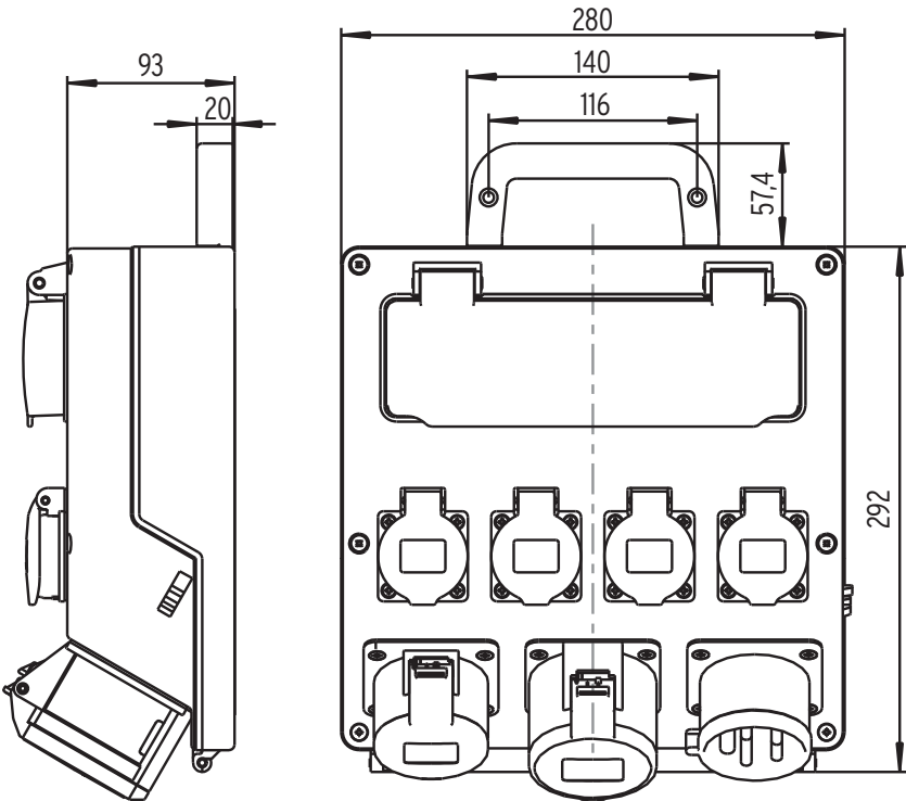
Abb. D: Gehäusemaße
