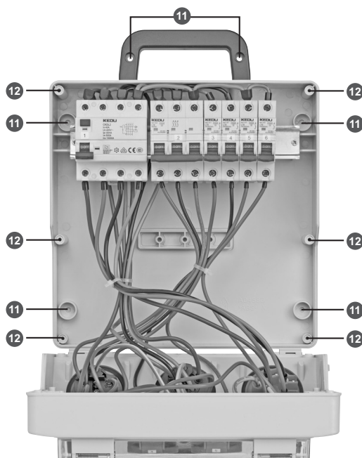
Fig. B: Exempel på väggfördelare 32 A
