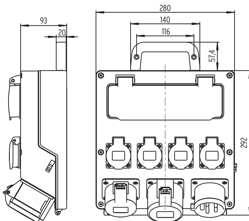
Fig. D: Kåpens dimensioner
