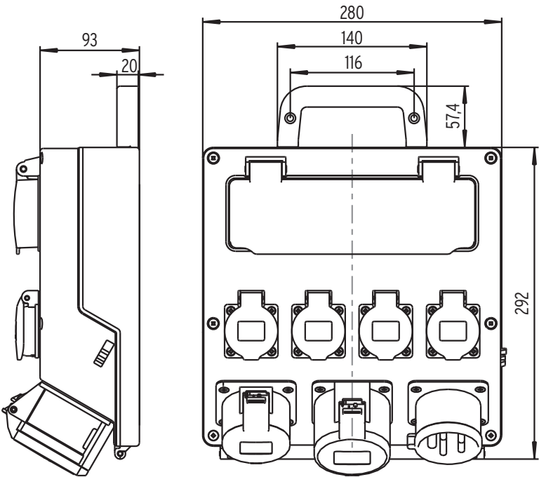
Рис. D: Размеры корпуса
