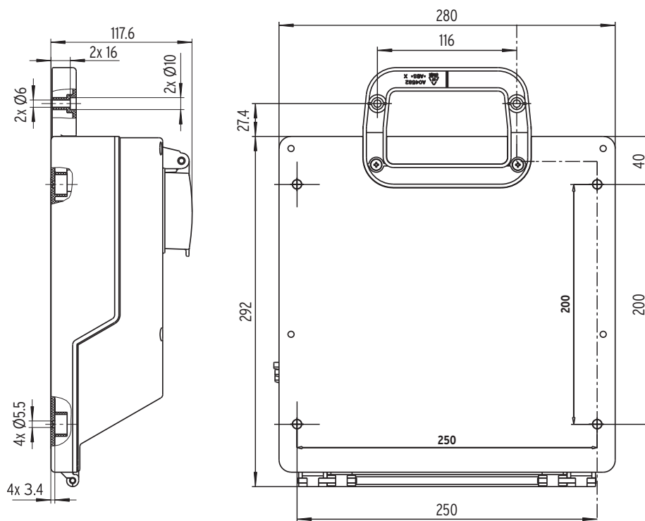
Abb. C: Bohrmaße
