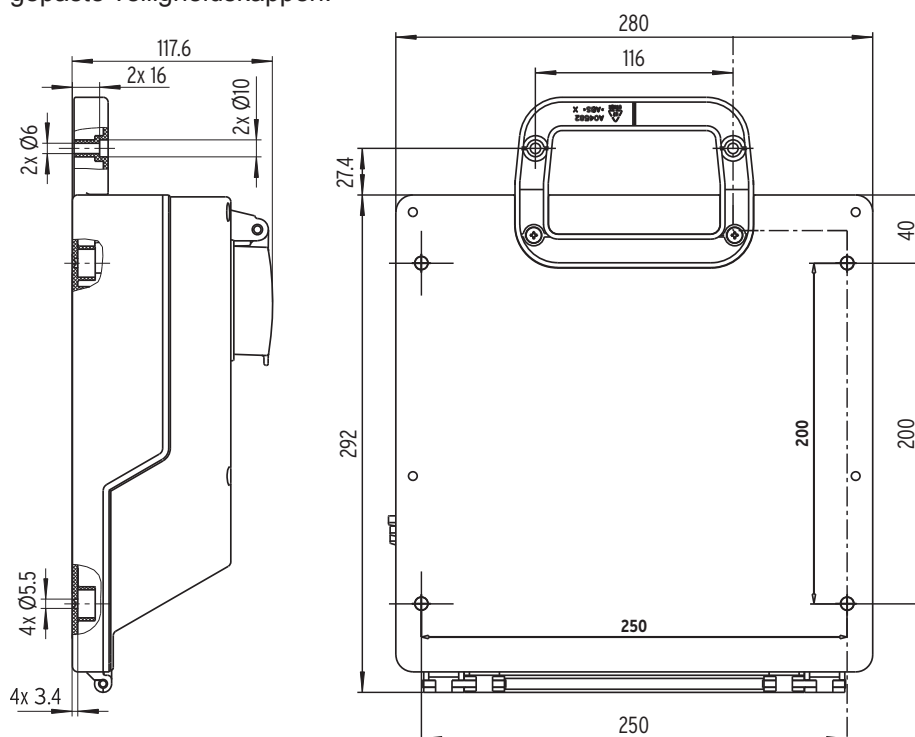
Afb. C: Boorafmetingen
