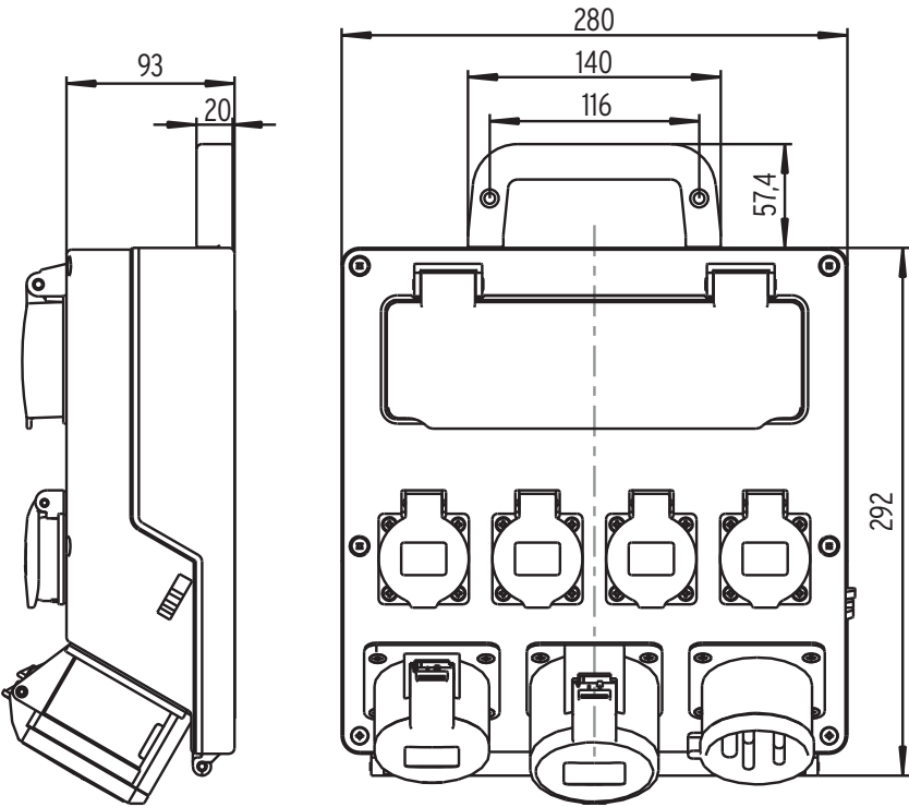
Afb. D: Afmetingen behuizing
