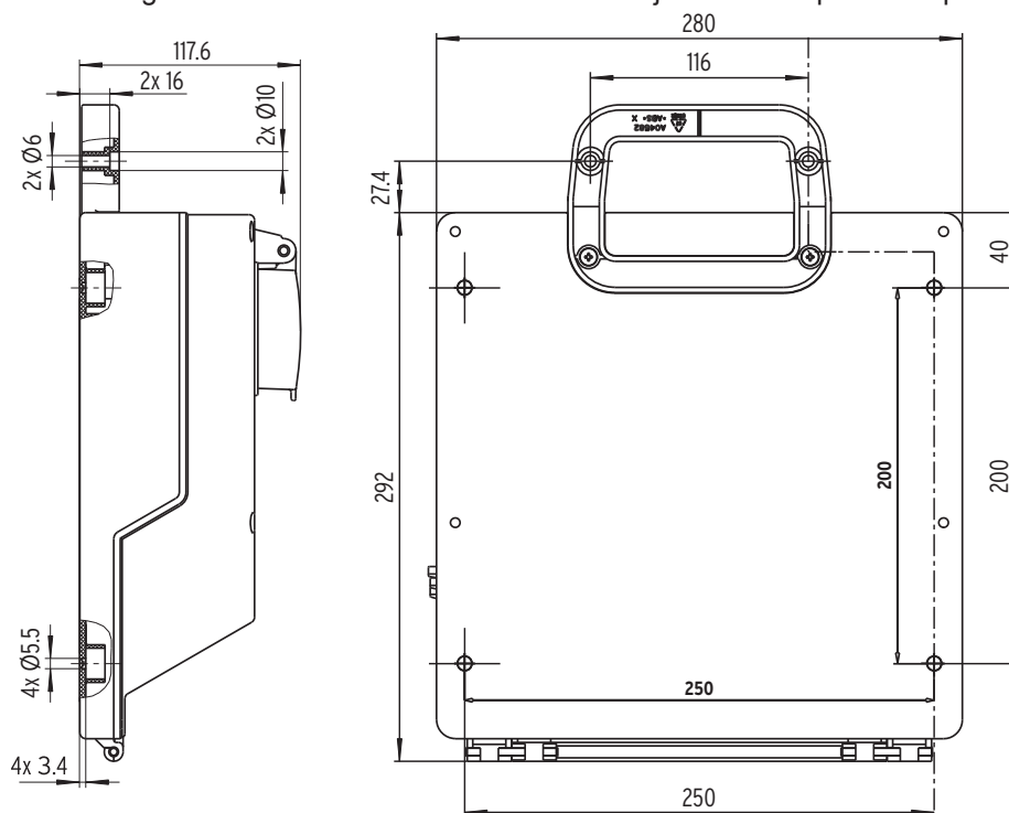
Fig. C: Perforación
