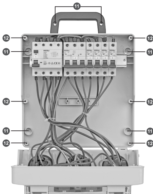
Abb. B: Beispiel Wandverteiler 32A
