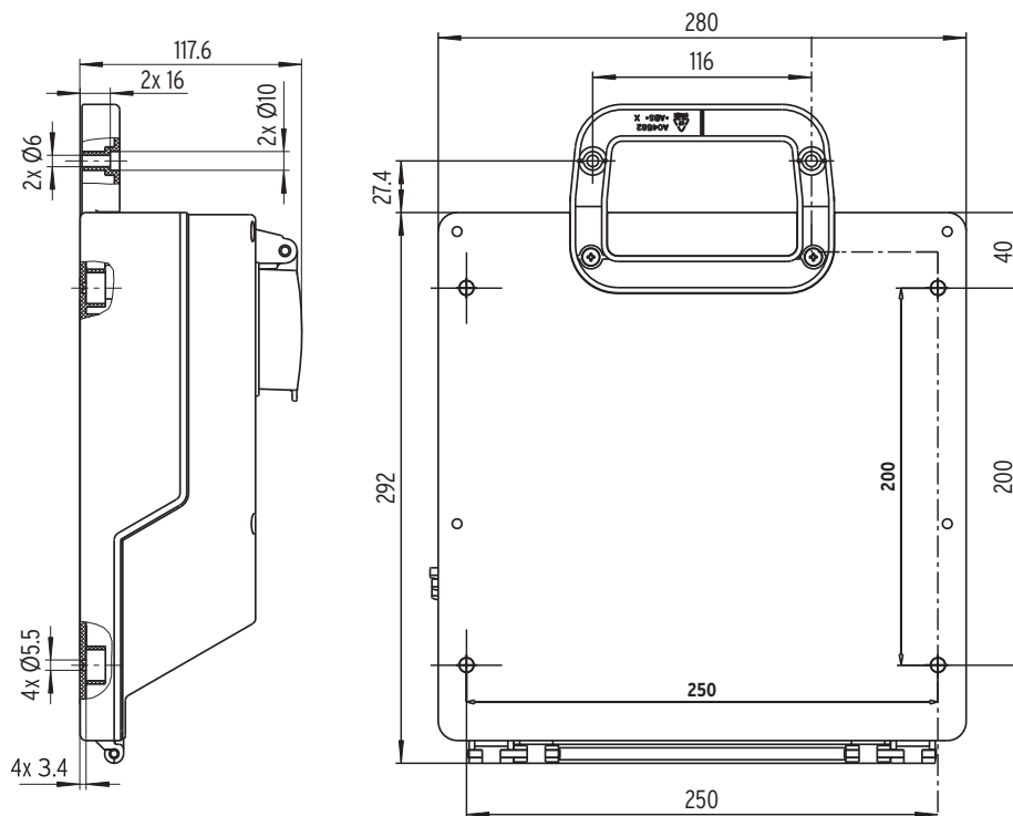
Fig. C: Borrmått
