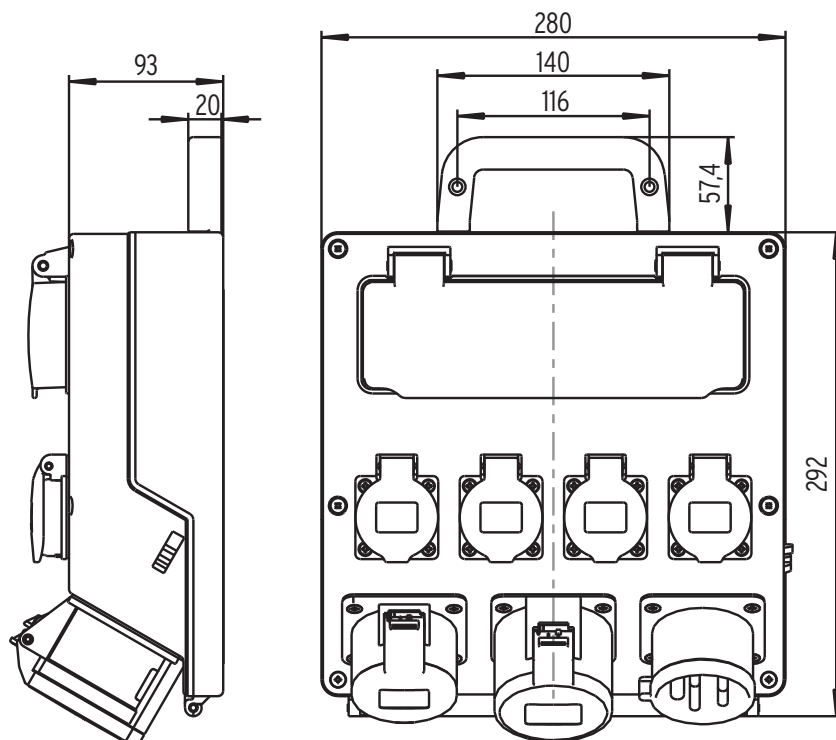
Kuva D: Kotelon mitat
