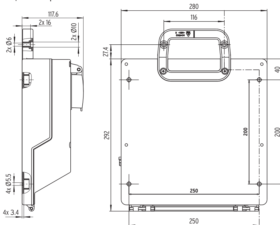
Рис. С: Размеры под расточку
