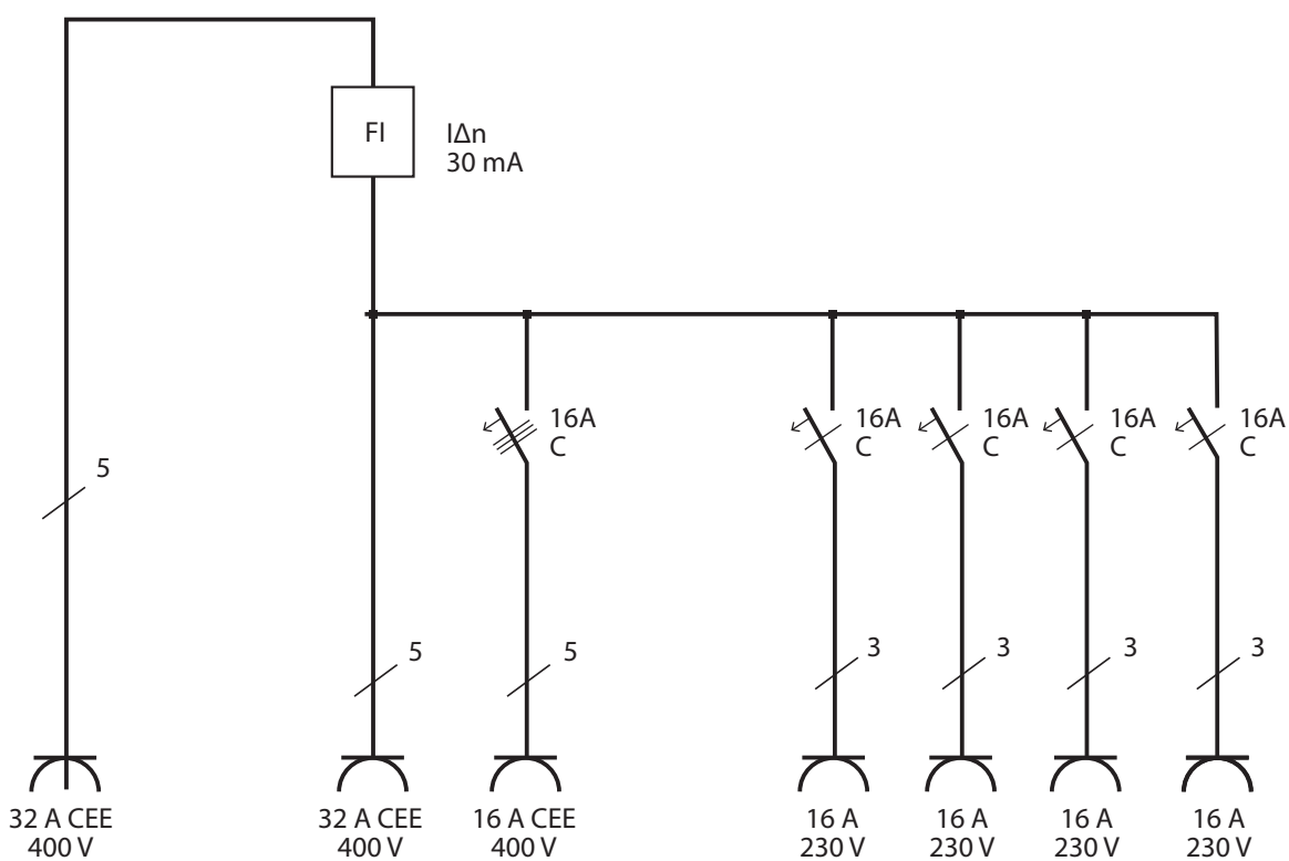
Fig. F: Vægfordelare WV 4/32A IP44
