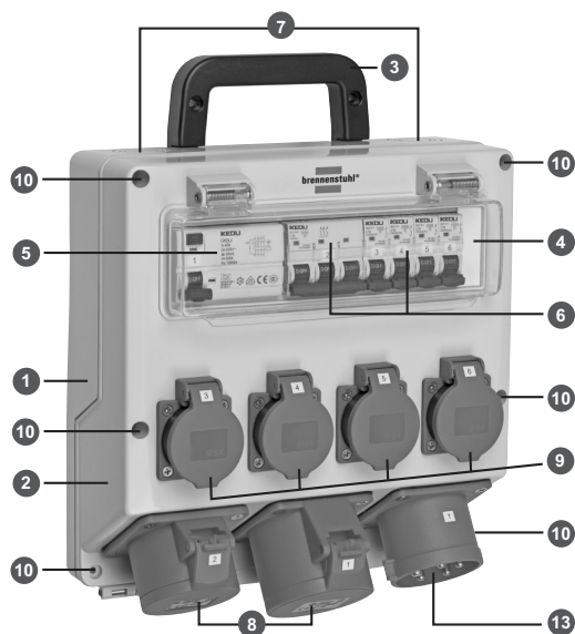
Fig. A: Exempel på väggfördelare 32 A
