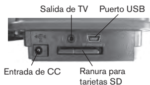
Fig. 1: Conexiones
