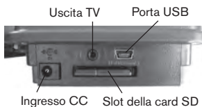
Fig. 1: Connessioni
