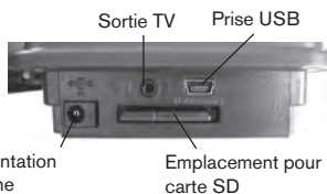
Fig. 1: Connexions
