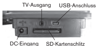
Abb. 1 : Anschlüsse
