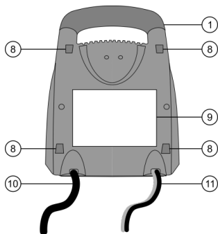
Afbeelding 2: achterzijde
