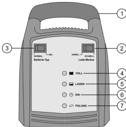
Bild 1: Ansicht Vorderseite
