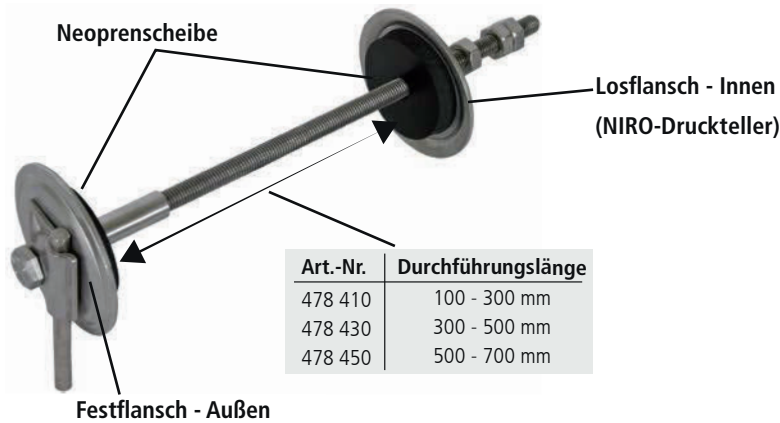
Bild 1 Wand- / Erderdurchführung
