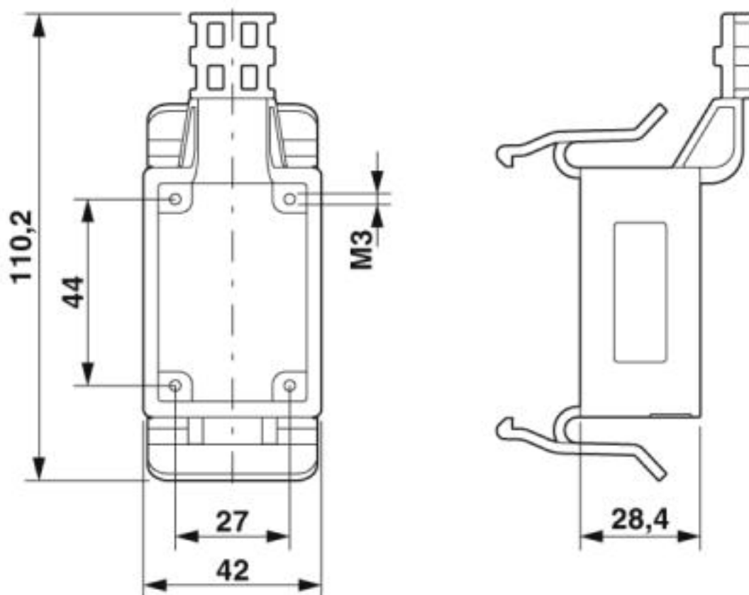
Maßzeichnung
