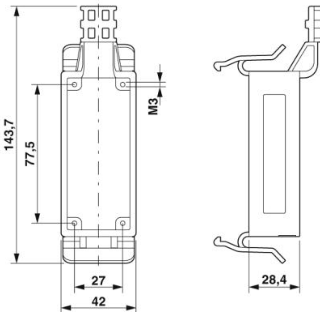
Maßzeichnung
