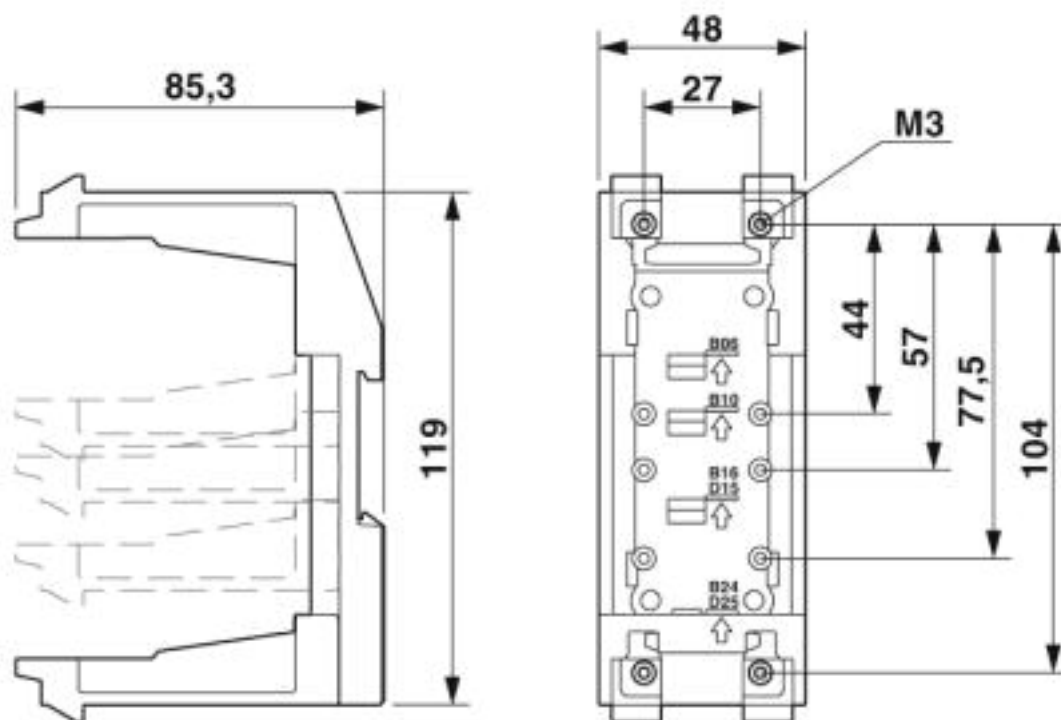
Maßzeichnung
