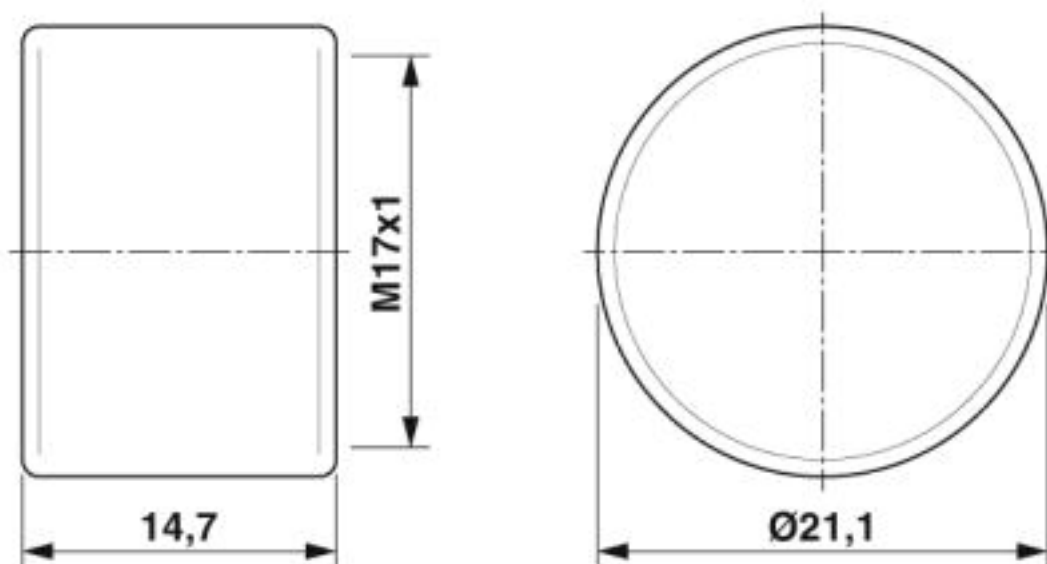
Maßzeichnung
