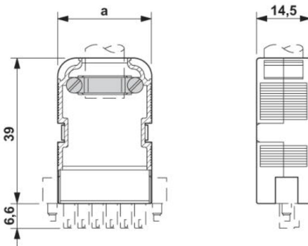
Maßzeichnung
