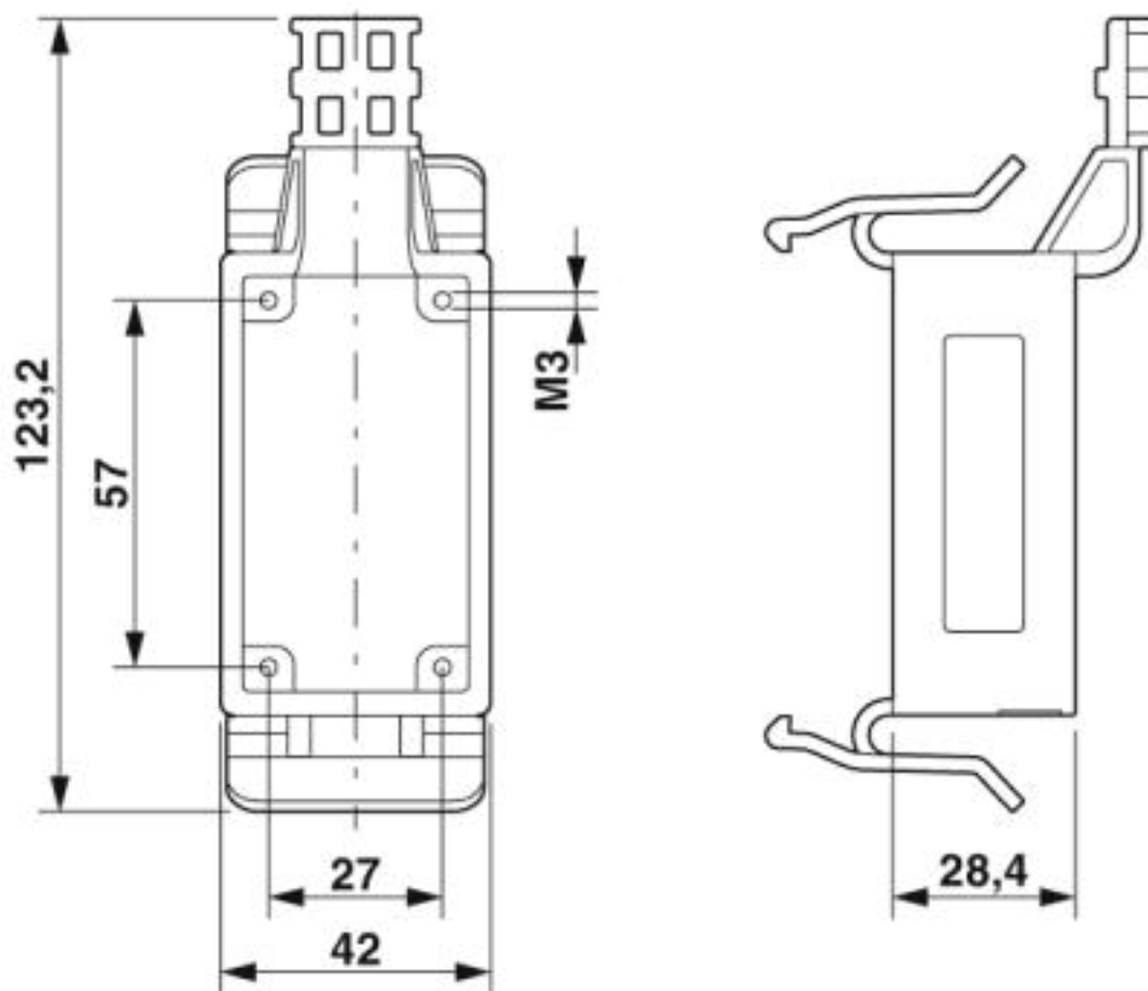
Maßzeichnung
