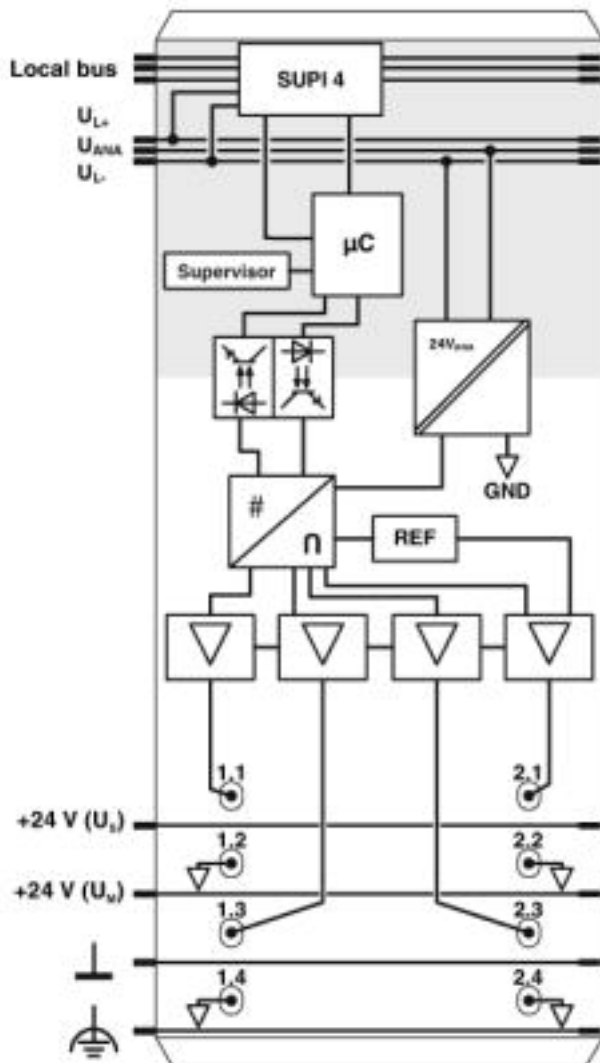
Interne Beschaltung der Klemmpunkte
