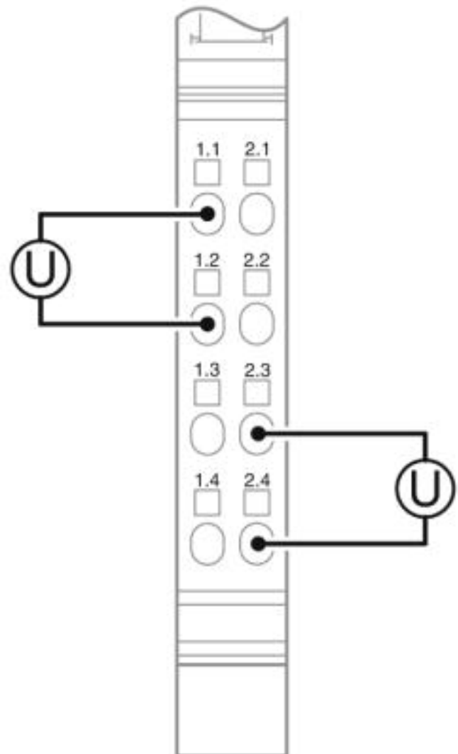
Anschluss der Aktoren
