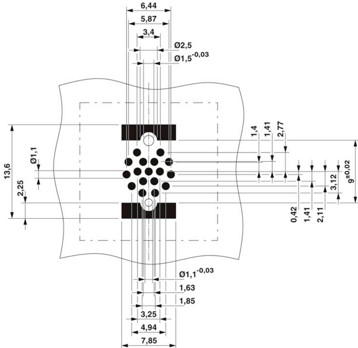
Bohrplan
