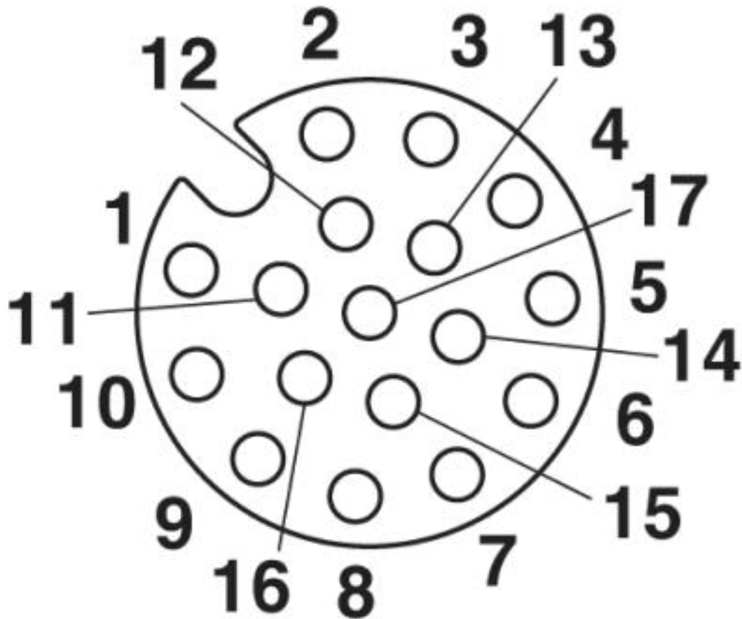
Polbild Buchse M12, 17-polig, A-kodiert, Ansicht Buchsenseite
