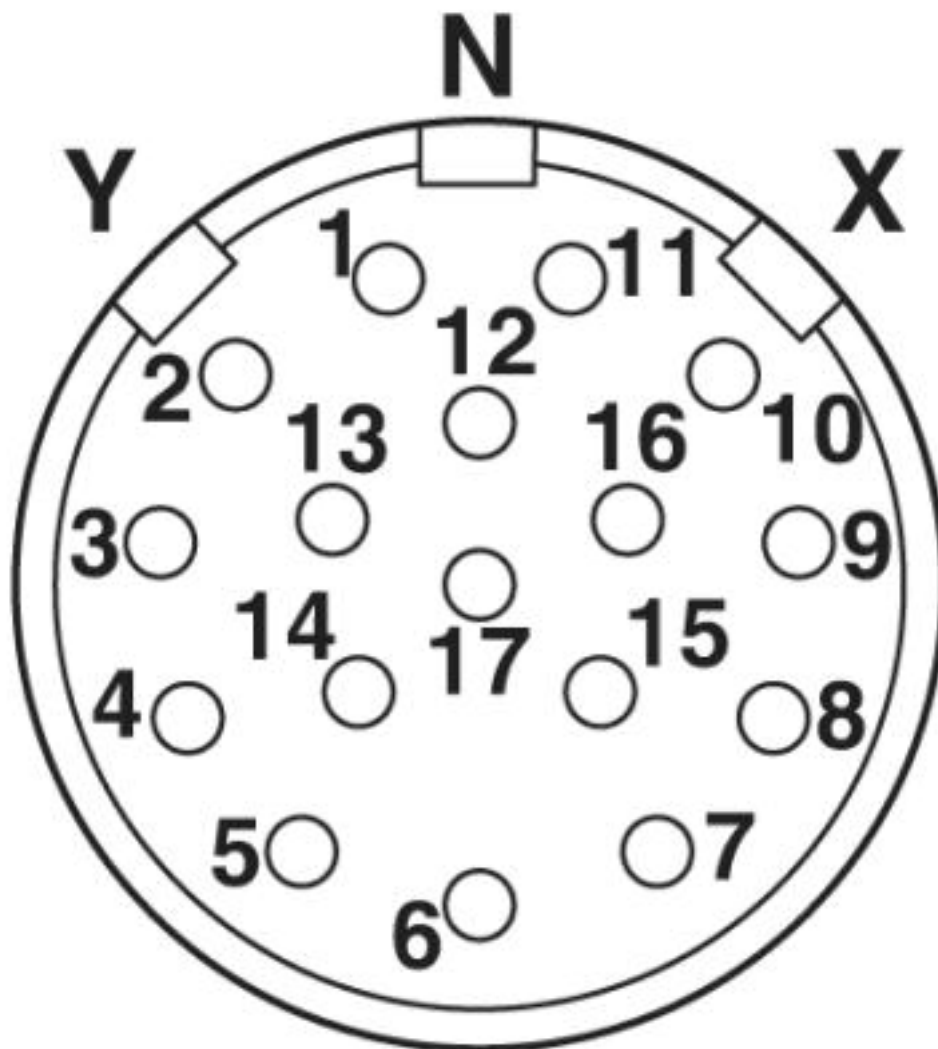
Schemazeichnung
