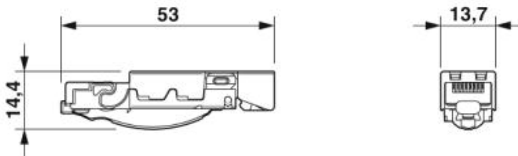
Maßzeichnung
