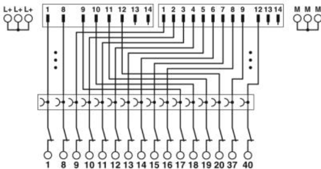
Schaltplan
