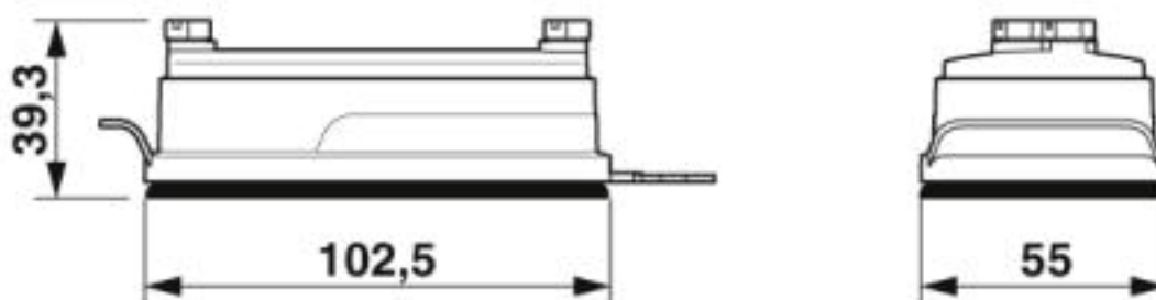
Maßzeichnung
