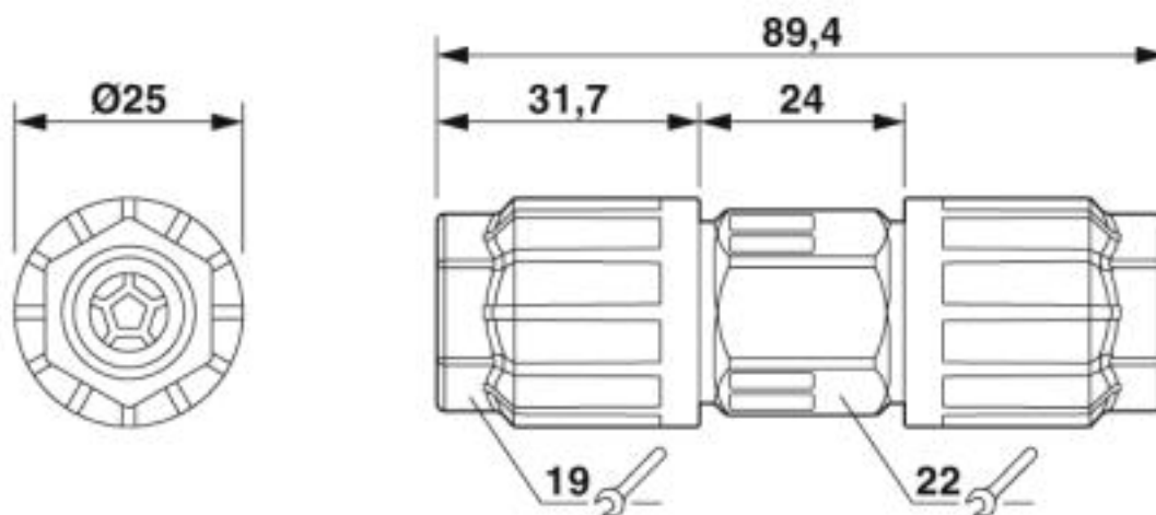
Maßzeichnung
