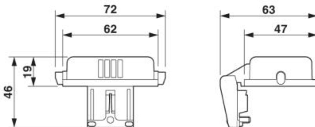
Maßzeichnung
