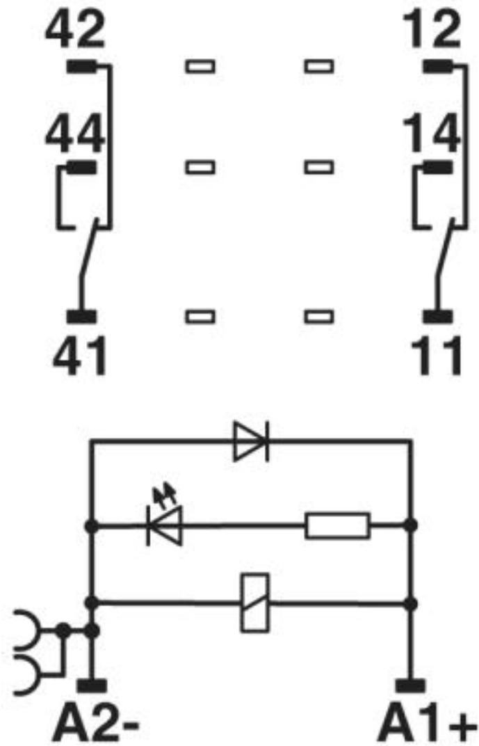
Schaltplan
