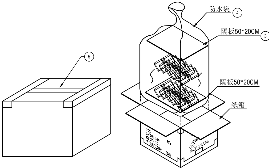
68PCS/CTN (580*230*230mm) 一排34pcs 上下兩排
