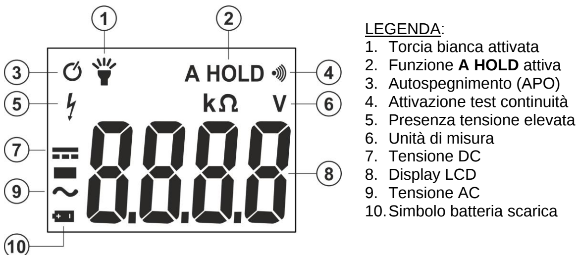
Fig. 2: Descrizione dei simboli a display
