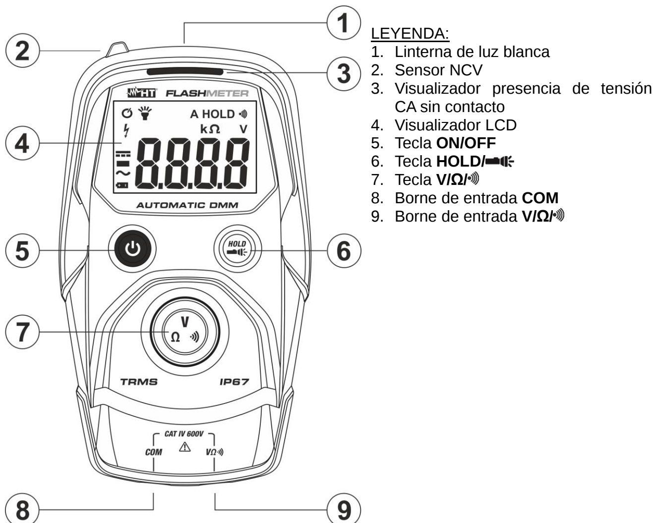
Fig. 1: Descripción del instrumento
