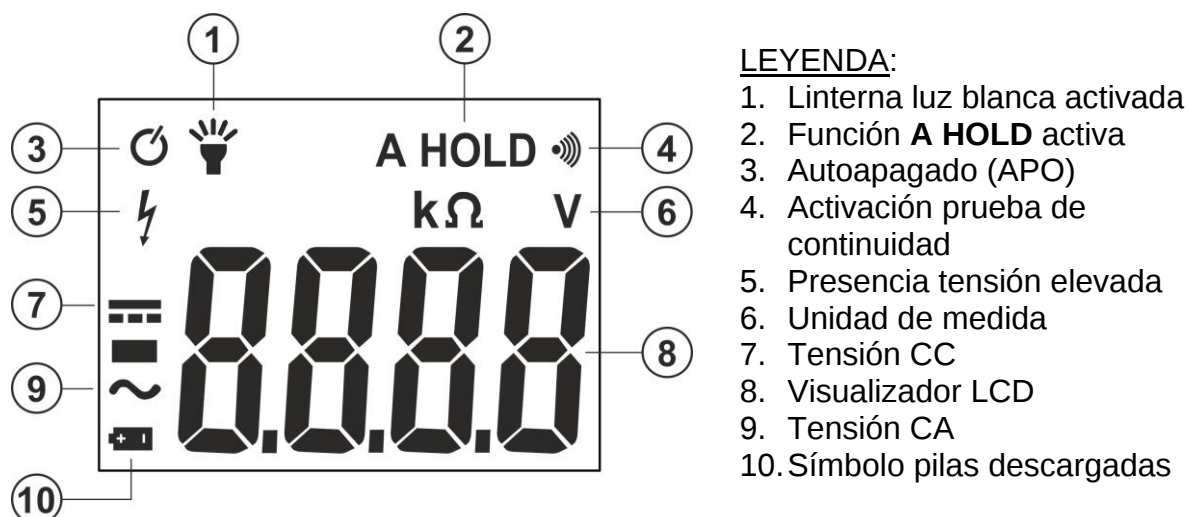
Fig. 2: Descripción de los símbolos en pantalla
