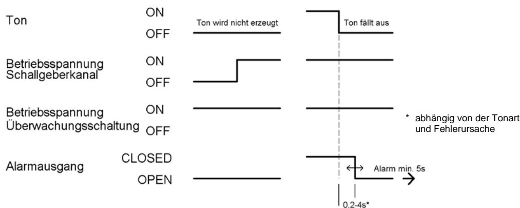
Abb. 8 Funktionszeitdiagramm bei Fehler
