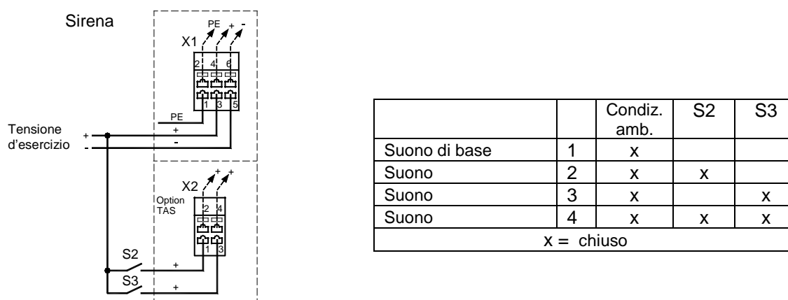
Fig. 10 Assegnazione delle connessioni, opzione TAS
