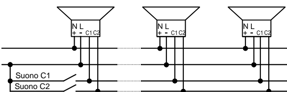
Esempio per comando DC "-"
