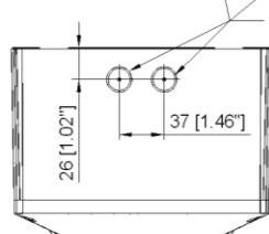
PA 10/ PA 20
