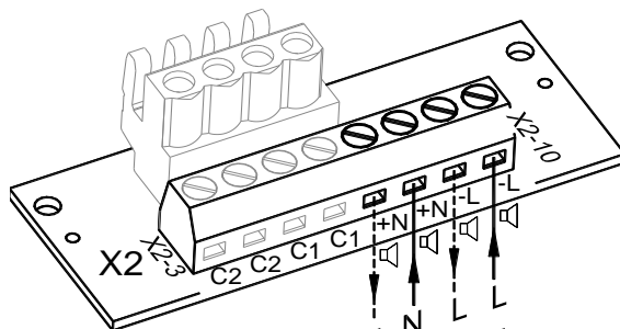
Подключение рабочего напряжения
