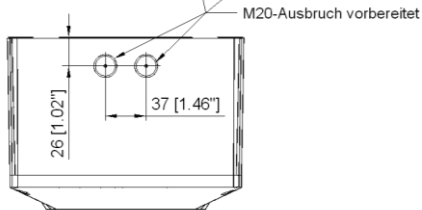
PA 10/ PA 20
