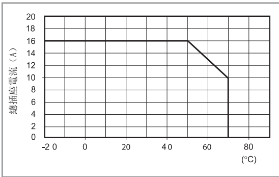
L 95 - 總插座電流與環境溫度
