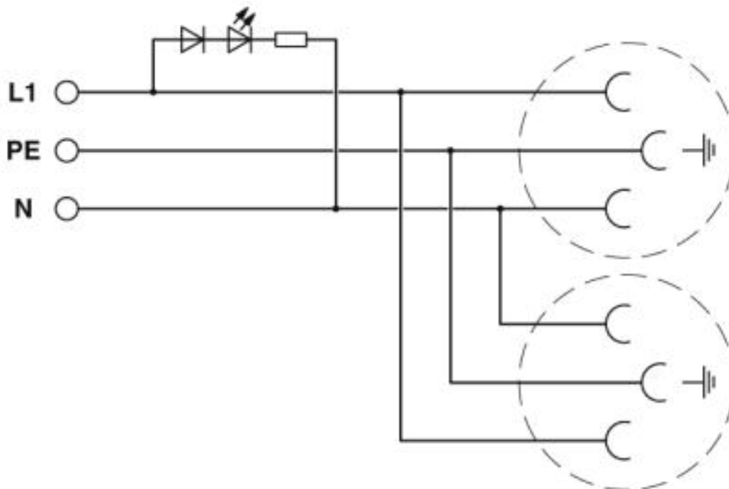
Schaltplan
