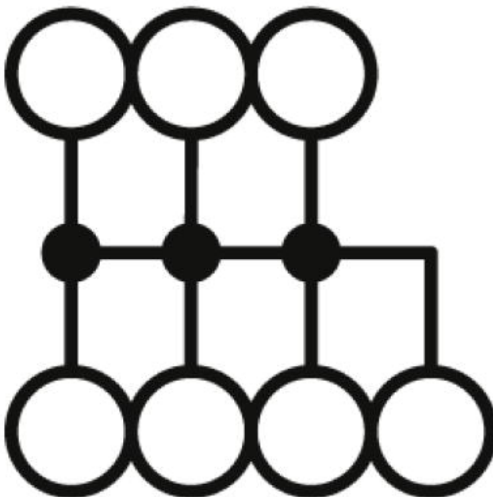
Schaltplan
