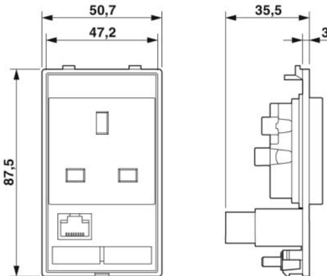
Maßzeichnung
