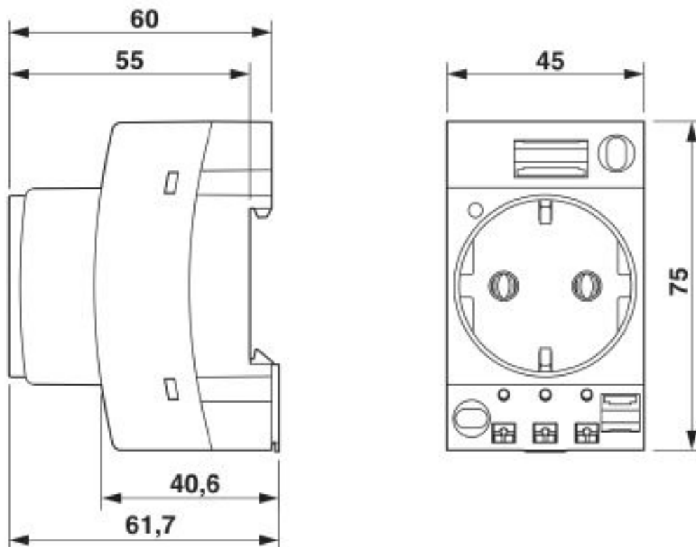
Maßzeichnung
